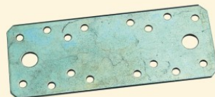
Пластина крепежная 180x65x2,0
