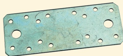
Пластина крепежная 210x90x2,0
