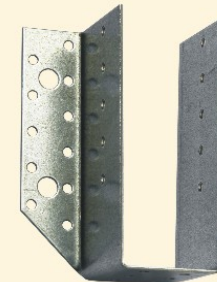
Опора бруса раскрытая 140x76x50x2,0 140x76x100x2,0
